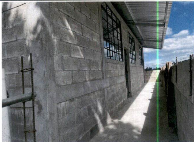
Foto 1: MEJORAMIENTO DE AULA TIPO PÓRTICO CON LÁMINA TROQUELADA CALIBRE 26
